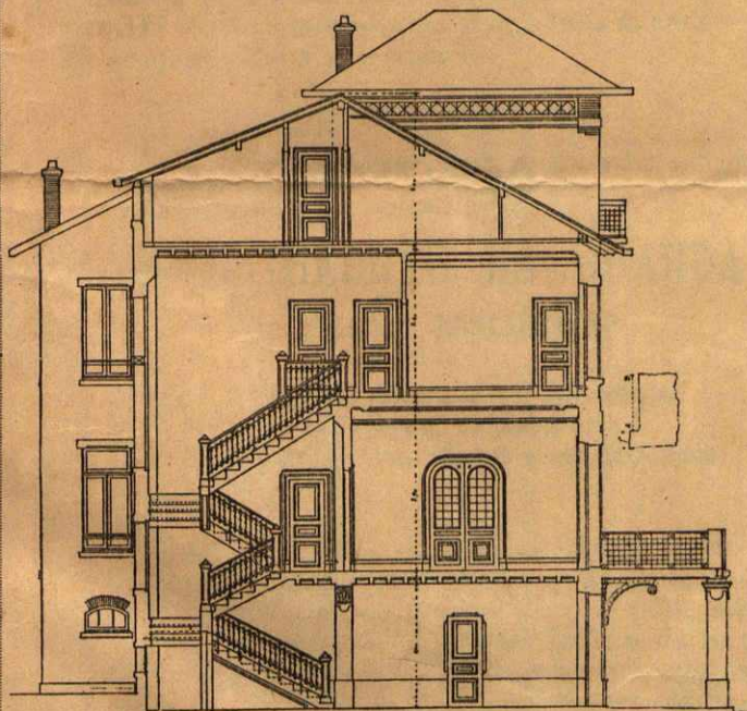
CORTE LONGITUDINAL
